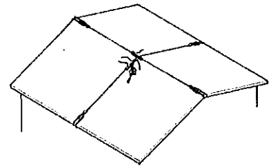
けらばに近づく場合は、親綱固定ロープによる補強を行う
