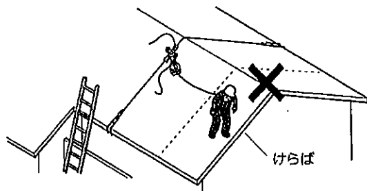
けらばには近づかない
