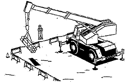
移動式クレーンによる荷のつり上げの際の措置の例
