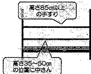
単管足場の場合の手すり等
