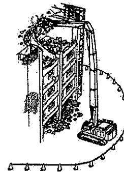
特定解体用機械であるコンクリート大割圧碎機による解体時の措置の例
