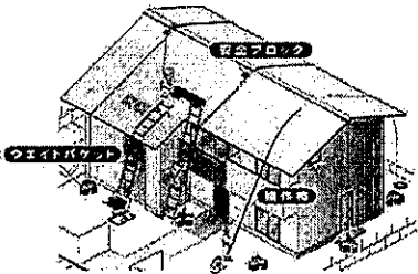
屋根：建物からの墜落防止工法（地上からの鰐網設置先行工法）
