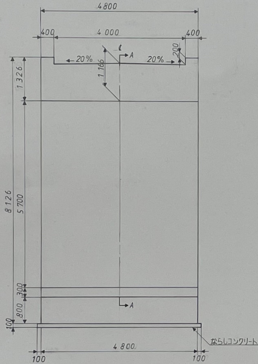
正面図
