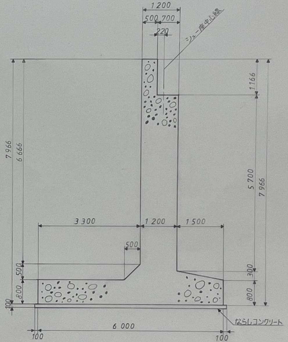
断面図 A-A
