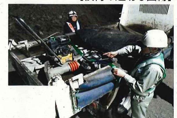
【積荷の適切な固縛】
