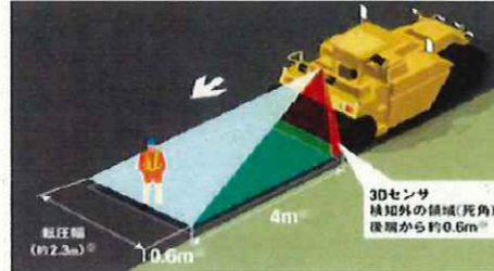
【センサーによる接触防止】
