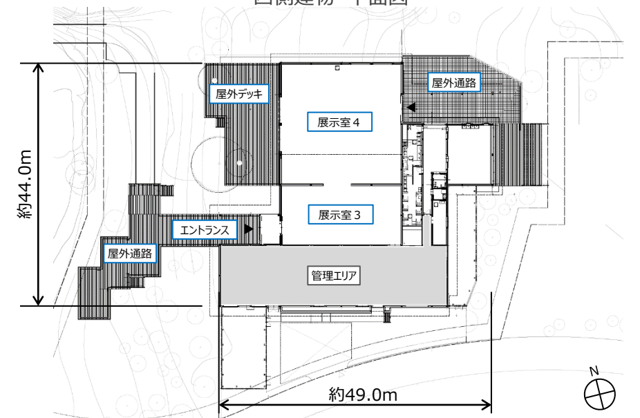
東側建物 平面図
