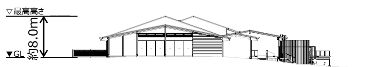
西立面図
